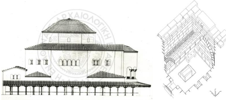
Σχέδιο με όψη του Οκταγώνου (αριστερά) και του εσωτερικού του παλιότερου ταφικού ηρώου (δεξιά) (Πελεκανίδης, Σ. 1972, Ανασκαφή Φιλίππων, ΠΑΕ, 74, εικ. 1 και Γούναρης, Γ. 1990. Το βαλανείο και τα βόρεια προσκίσματα του οκταγώνου Φιλίππων, σχ.17)
