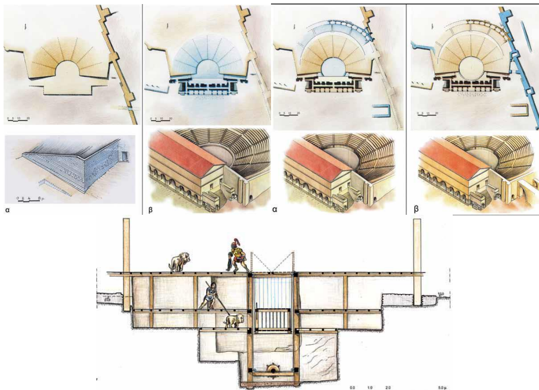
Οι διαφορετικές φάσεις του θεάτρου και το σύστημα ανύψωσης (Καραδέδος, Γ. 2012. Το αρχαίο θέατρο των Φιλιππων, 196-201)
